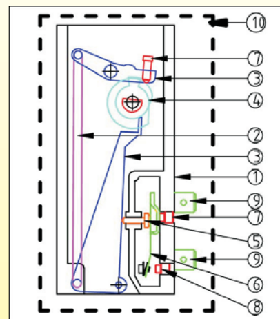
Diagrama esquemático
