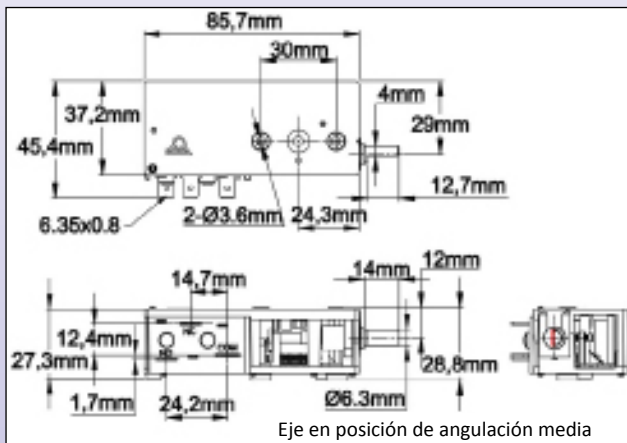
Eje en posición de angulación media
